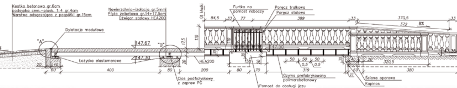
PRZEKRÓJ PODŁUŻNY W OSI KŁADKI
